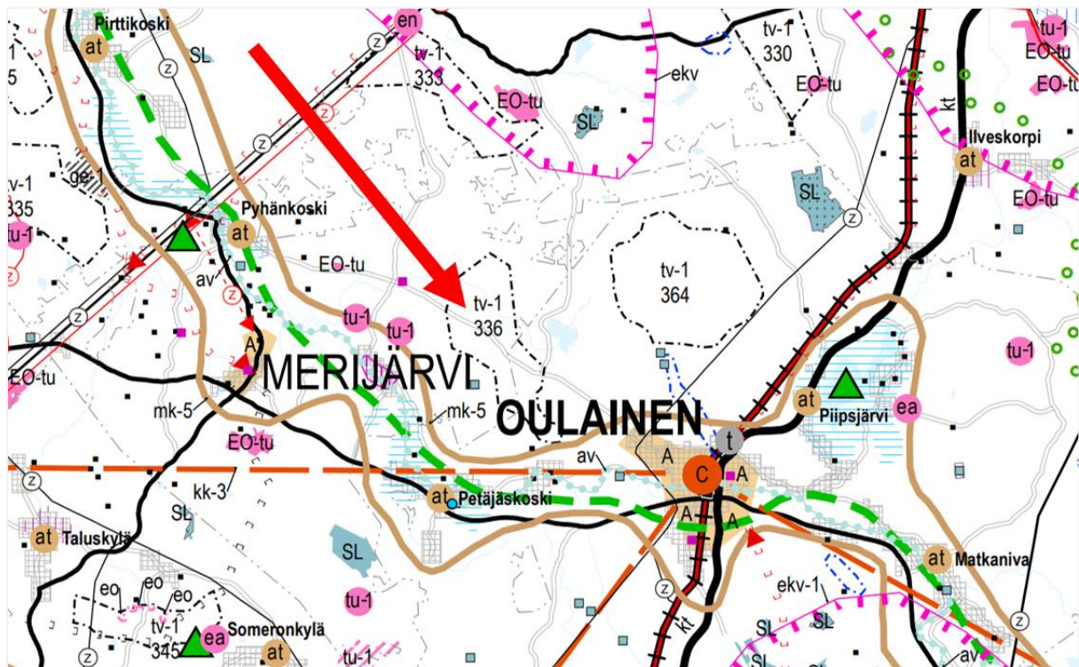
Kuva 6. Ote Pohjois-Pohjanmaan maakuntakaavojen yhdistelmäkartasta (18.1.2022). Suunnittelualueen likimääräinen sijainti merkitty punaisella nuolella. (Lähde: Pohjois-Pohjanmaan liitto)
