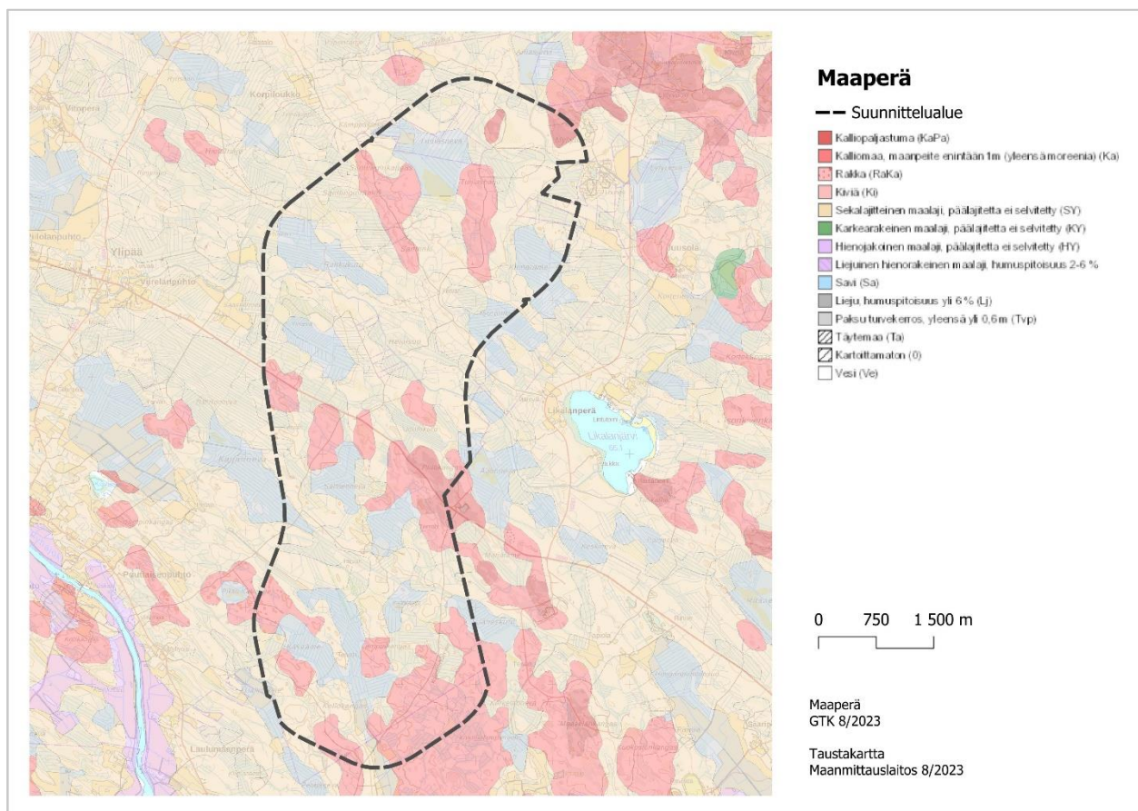
Kuva 3. Suunnittelualueen sijainti maaperäkartalla. (Lähde: Maaperä, GTK & Taustakartta, Maanmittauslaitos)
