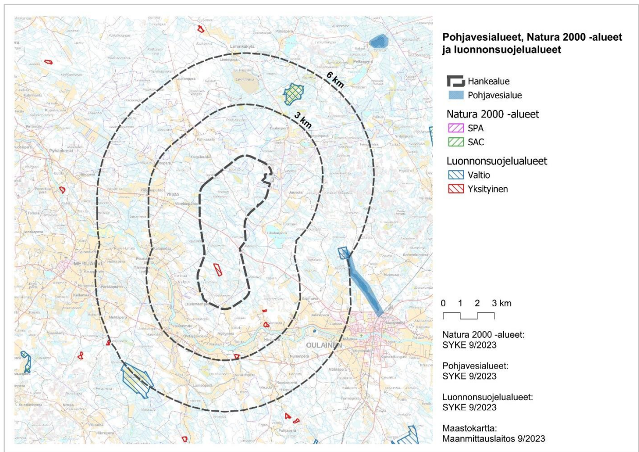
Kuva 4. Suunnittelualueen sijainti suhteessa Natura 2000 -alueisiin, luonnonsuojelu-alueisiin ja pohjavesialueisiin. Kartassa on osoitettu myös etäisyysvyöhykkeet suunnittelualueen rajasta. (Lähde: Natura 2000 -alue, luonnonsuojelualue ja pohjavesialue, SYKE)
