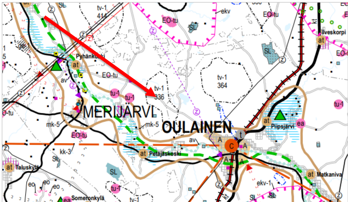
Kuva 10. Ote Pohjois-Pohjanmaan energia- ja ilmastovaihemaakuntaavan yhdistelmäkartasta (jossa ehdotusvaiheen merkinnät ja voimassa olevat maakuntakaavat näkyvät). Suunnittelualueen likimääräinen sijainti on osoitettu punaisella nuolella. (Lähde: Pohjois-Pohjanmaan liitto)
