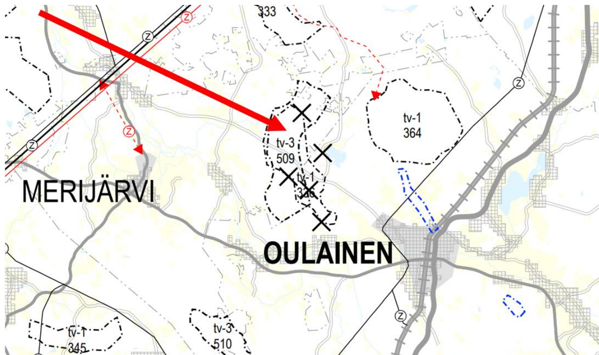
Kuva 7. Ote Pohjois-Pohjanmaan energia- ja ilmastovaihemaakuntaavan kaavaluonnoskartasta (21.6.2022). Suunnittelualueen likimääräinen sijainti osoitettu punaisella nuolella.
