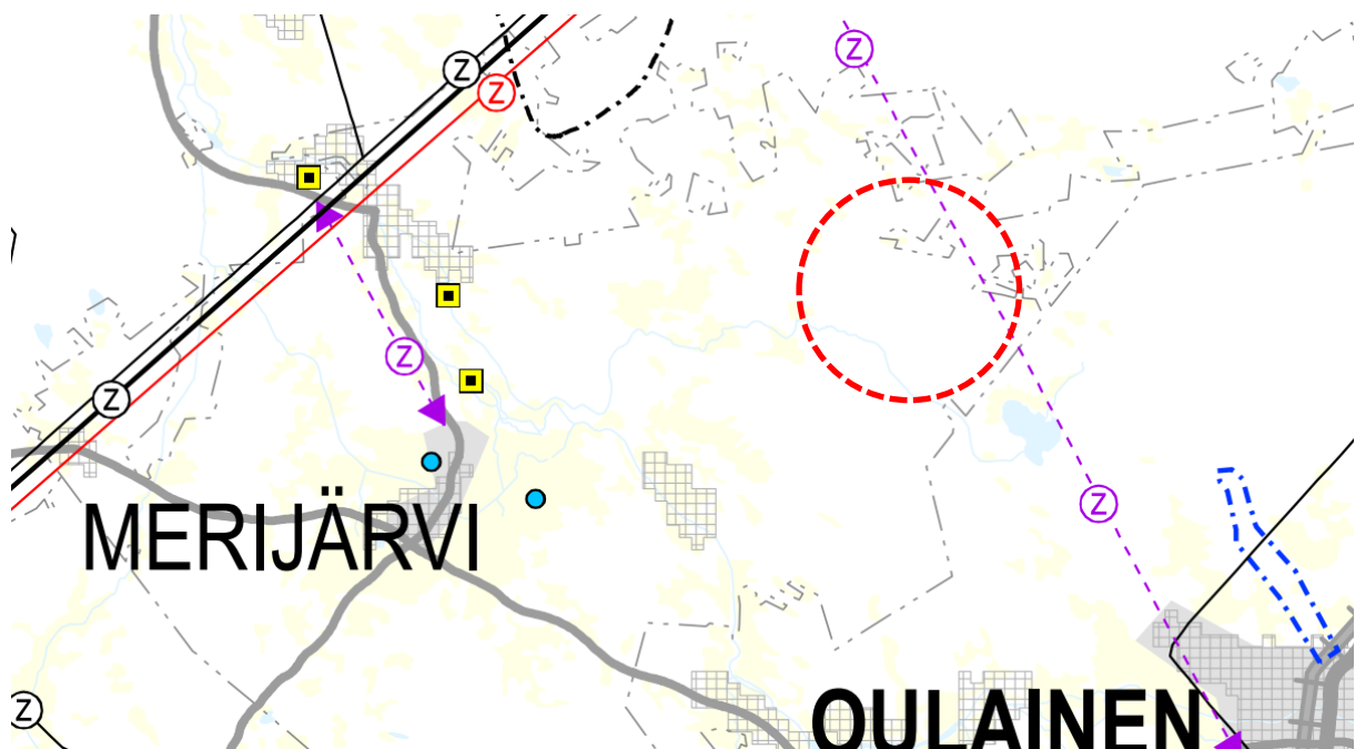
Kuva 8. Ote Pohjois-Pohjanmaan energia- ja ilmastovaihemaakuntaavan nähtävillä olevasta 2. kaavaehdotuskartasta (MKH 10.2.2025). Suunnittelualueen likimääräinen sijainti osoitettu punaisella katkoviivalla.
