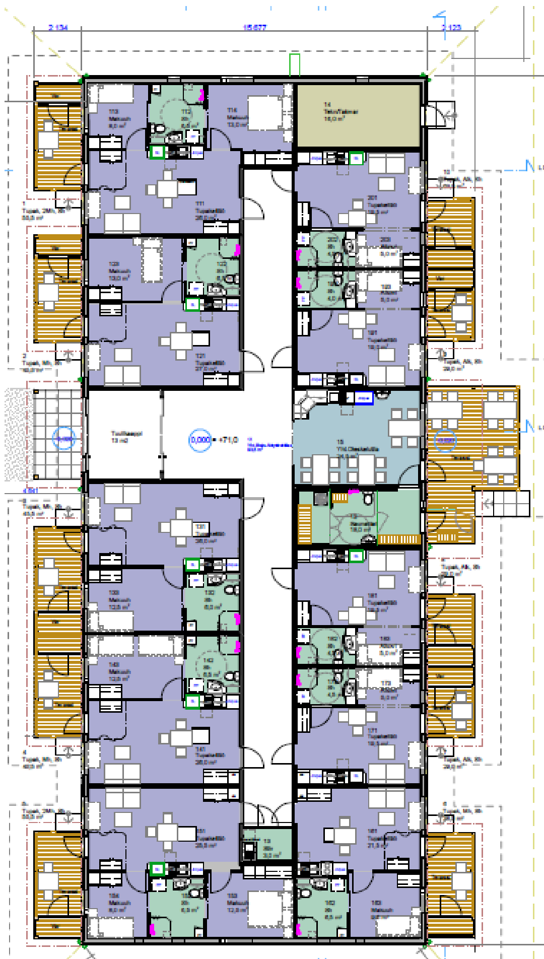
Pohjapiirustus
